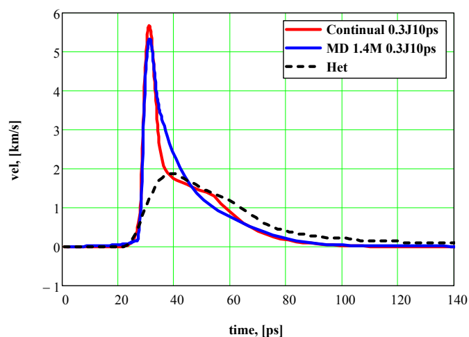
Рис. 1. Скорости фронта плавления, полученные при континуальном и МД моделировании.
