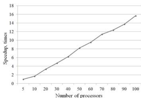
Рис. 1. Ускорение в зависимости от числа процессоров
