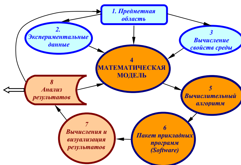
Рис.1 Схема вычислительного эксперимента.
