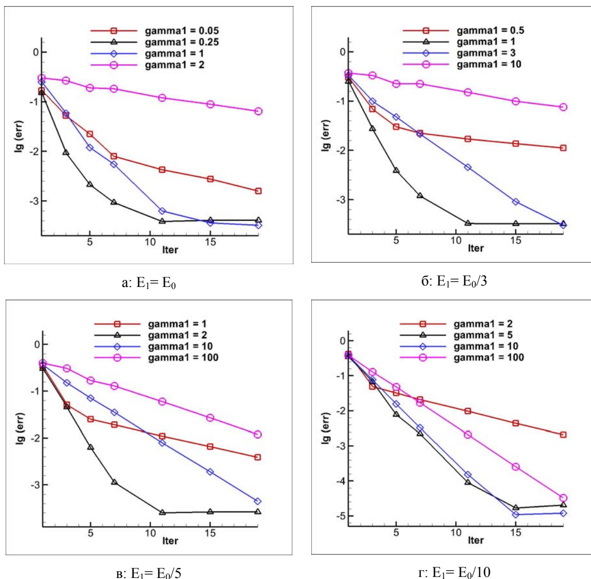
Рис. 3. Графики зависимости десятичного логарифма ошибки от номера итерации для расчетов 1.1-1.4
